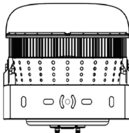
Side EPA: 0.333m 2 | 3.59ft 2
